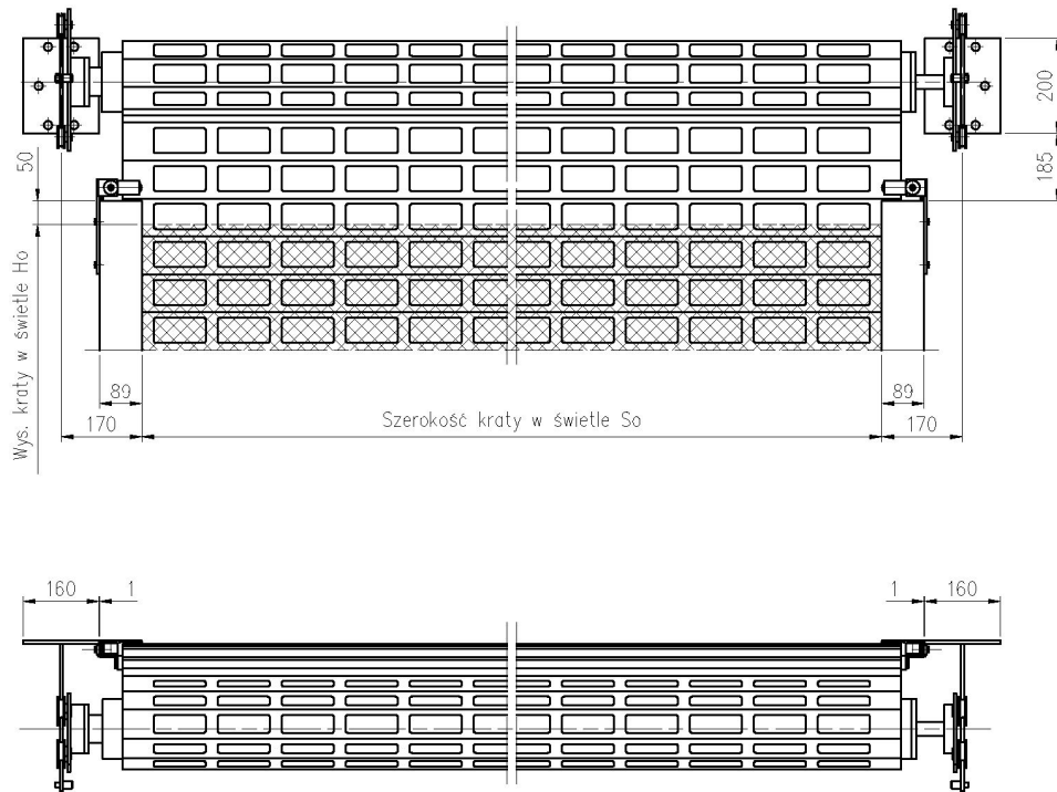
Rys. 3. Krata na konsoli KNB
