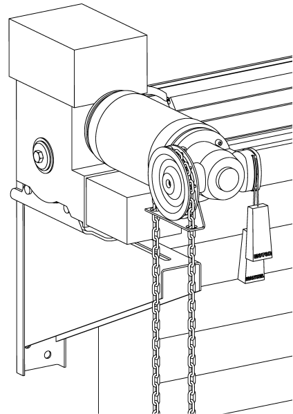
Rys.5. Napęd awaryjny łańcuchowy
