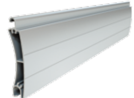
PE 55 | wysokość profilu: 55 mm grubość: 14 mm
